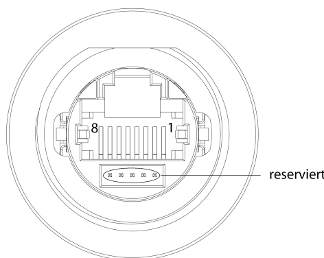
Abb. 5: PoE-Steckverbinder
