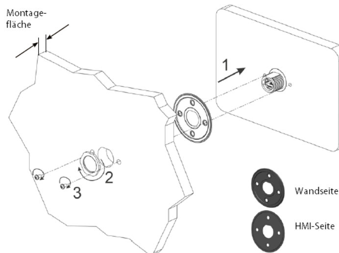
Abb. 4: Montieren TXF700
