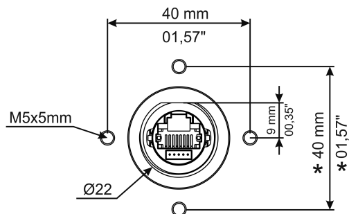
Abb. 6: PoE-Steckverbinder – Abmessungen
