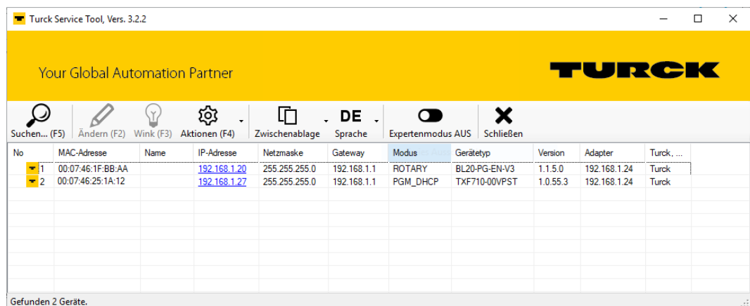
Abb. 10: Turck Service Tool – gefundene Geräte
