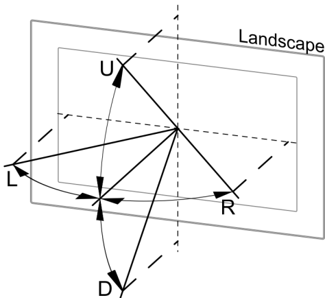
Abb. 13: Betrachtungswinkel
