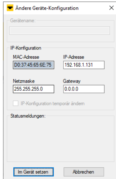
Abb. 11: Turck Service Tool – IP-Konfiguration ändern
