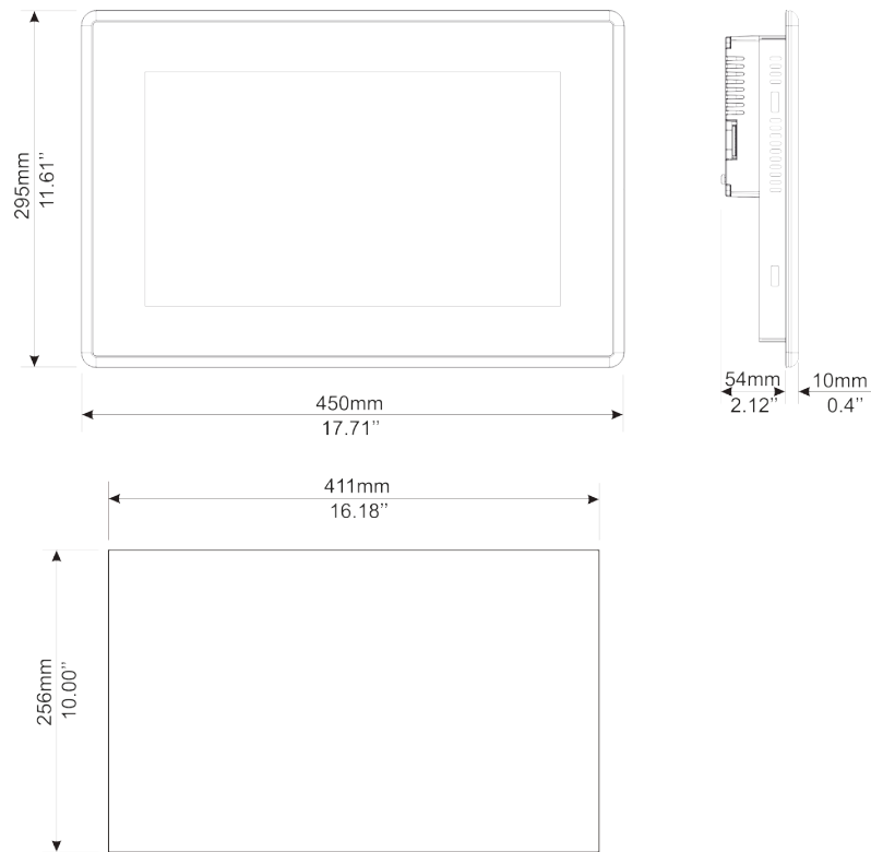
Abb. 4: Abmessungen – TX715FB
