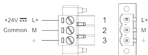
Abb. 11: Spannungsversorgungsstecker TX7...
