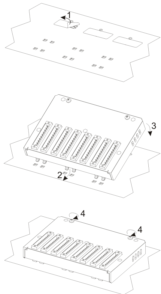
Abb. 8: Plug-in-Module montieren (z. B. TX-IO-XX03)
