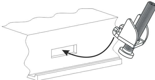
Abb. 6: Halteklammern einsetzen
