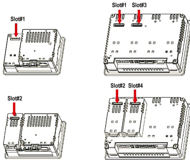
Abb. 13: Erweiterungssteckplätze für Plug-in-Module
