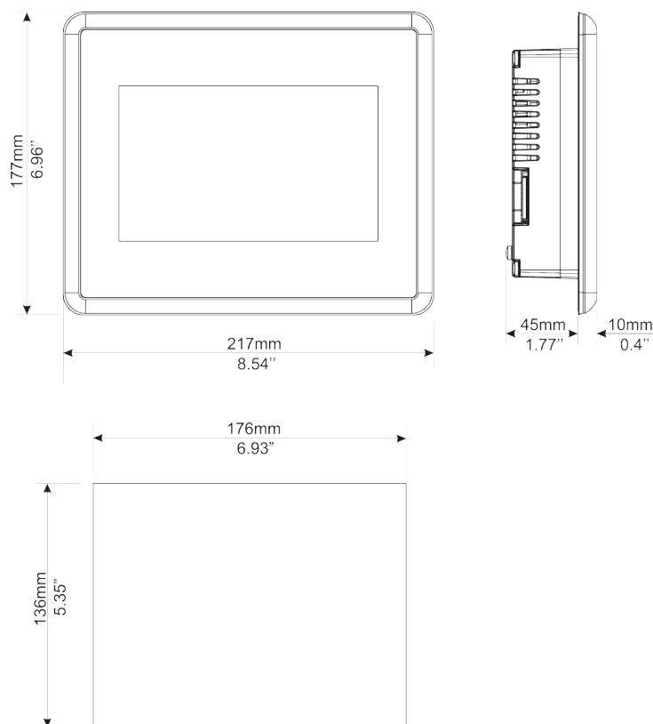
Abb. 3: Abmessungen – TX707FB
