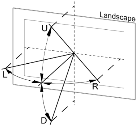
Abb. 20: Betrachtungswinkel
