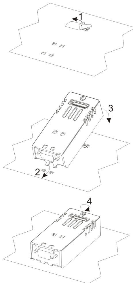
Abb. 7: Plug-in-Module montieren (z. B. TX-CAN, TX-IO-DX06)
